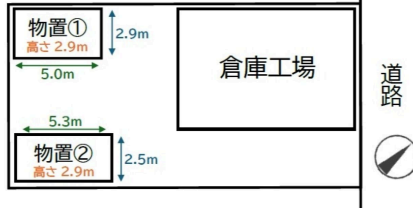
配置図
